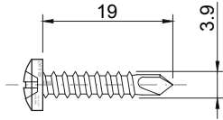
290472 PARAF. AT/PF CQ 3.9x19 A2
