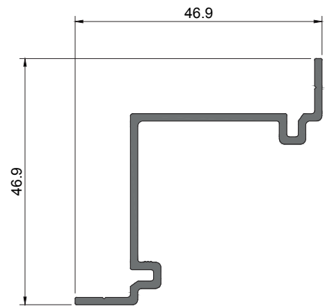
SQ 02 Perfil para cantos Angles profile | Profilé pour angles
