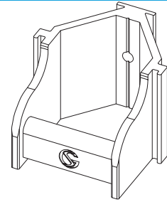
230283 SUPORTE EM POLIAM. VO P/PAINEL Material: Poliamida 6 V0 (material Ignifugo)
