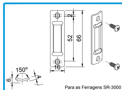
202083 Para as Ferragens SR-3000 CONTRA-FECHO 2070.861
