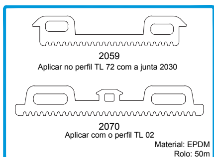
208907 JUNTA REMATE PAREDE 2059 208287 JUNTA REMATE PAREDE 2070
