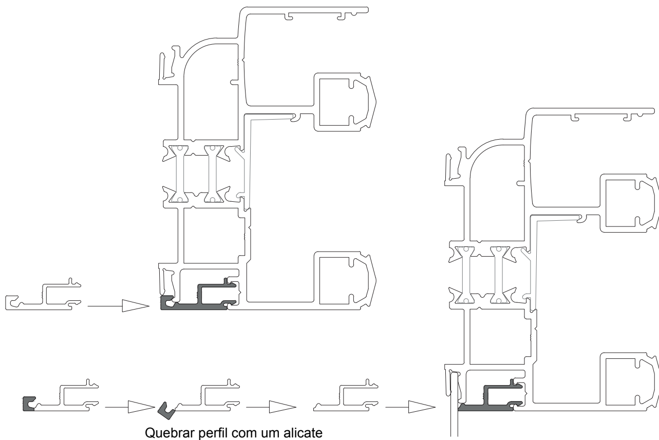
REMATE LATERAL TL 30 MEDIDA DE CORTE = H-38mm
