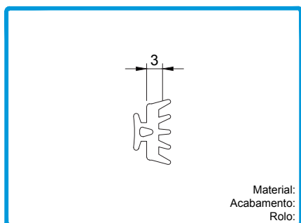
208289 JUNTA DE BATENTE 2055
