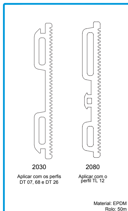
208208 JUNTA REMATE PAREDE 2080 208388 JUNTA REMATE PAREDE 2030
