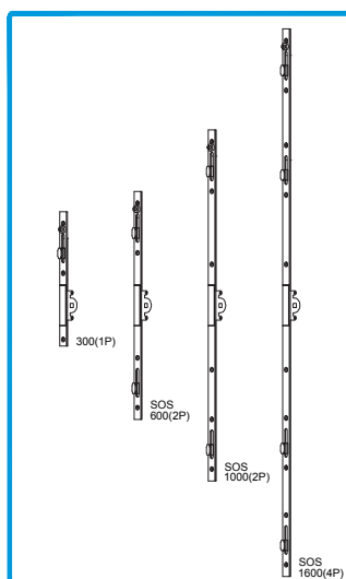
211205 FERR. MULTIPONTO 300 (1P) 211191 FERR. MULTIPONTO SOS 600 (1P) 211192 FERR. MULTIPONTO SOS 1000 (2P) 211193 FERR. MULTIPONTO SOS 1600 (4P)
