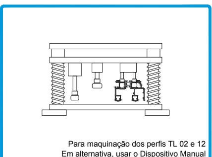
408004 CORTANTE AM CORRER Para maquinação dos perfis TL 02 e 12 Em alternativa, usar o Dispositivo Manual
