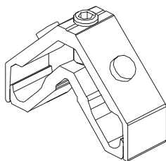
Para os perfis TL 05, 55, 41, 64, 72, 73 e 74 Maquinização com o cortante para esquadros EURO2000
