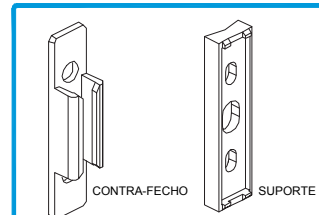
202098 CONTRA-FECHO MP 300 (1P) 230303 SUPORTE P/C.-FECHO MP 300 (1P)
