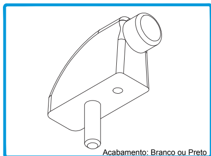
214164 BATENTE TOPEHSN Acabamento: Branco ou Preto
