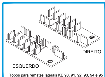
212223 CONJUNTO TOPOS INFERIORES RENOVATIO
