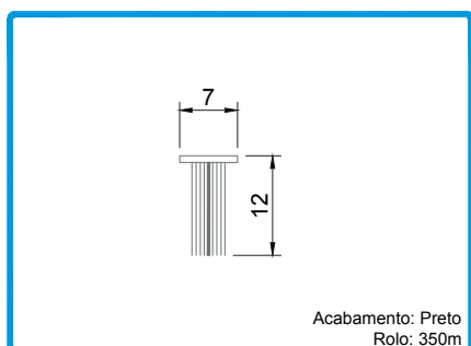
208593 PELÚCIA 7x12 S-FINE CINZA
