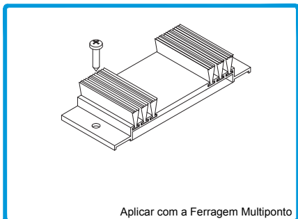
213285 CORTA VENTO AM/TL 02
