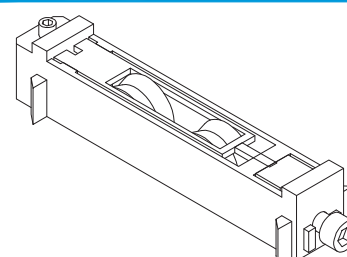
Carrinho de 2 roda regulável, de agulhas Resistência por folha com 2 carrinhos: 100Kg
