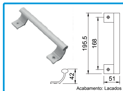
201375 ASA PARA FECHO LATERAL 2080
