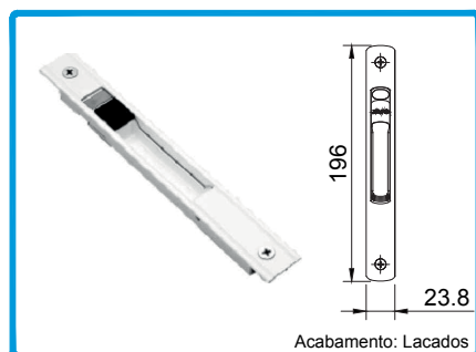
201478 FECHO LAT. MANUAL 2070 201470 FECHO LAT. MANUAL 2071
