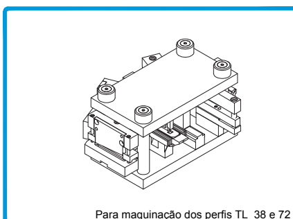
408033 CORTANTE SÉRIES SA2000+AT2100 Para maquinação dos perfis TL 38 e 72
