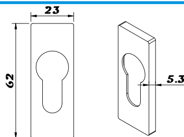
220196 ESPELHO ALUMÍNIO 23MM P/ SEGREDO
