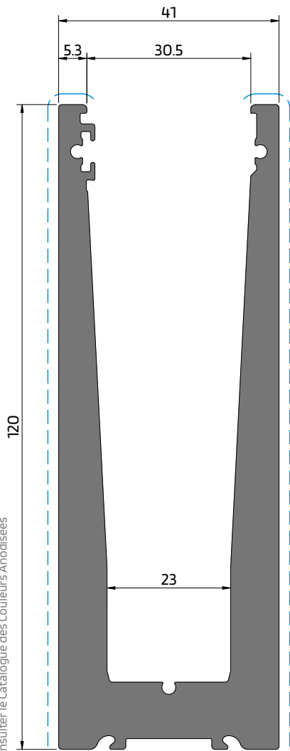
AV 03 Sem furações Without milling Sans fraisage
