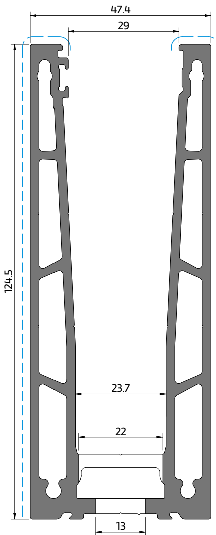
AV 24 Com furações inferiores With inferior milling Avec fraisage inférieur
