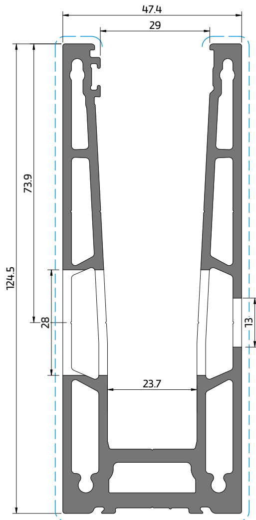
AV 25 Com furações laterais With lateral milling Avec fraisage latérale
