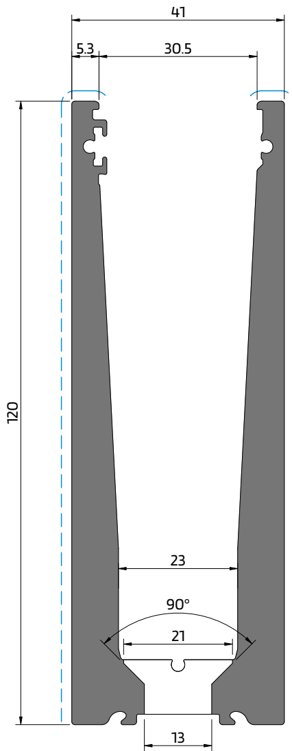
AV 13 Com furações inferiores With inferior milling Avec fraisage inférieur
