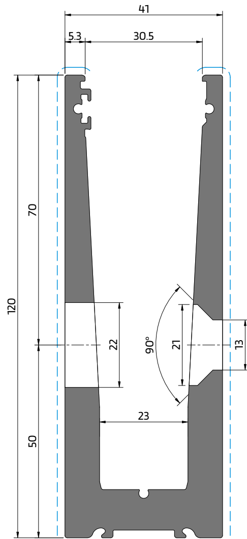
AV 14 Com furações laterais With lateral milling Avec fraisage latéral
