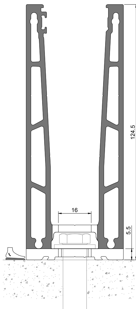
AV 30 ** Com furações inferiores e drenagem With inferior milling and drainage Avec fraisage inférieur et drainage
