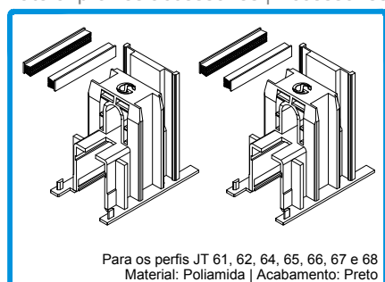
212199 CONJ. TOPOS LAT. JT N°1
