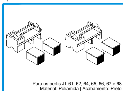
212230 CONJ. TOPOS INTERIORES LAT. JT
