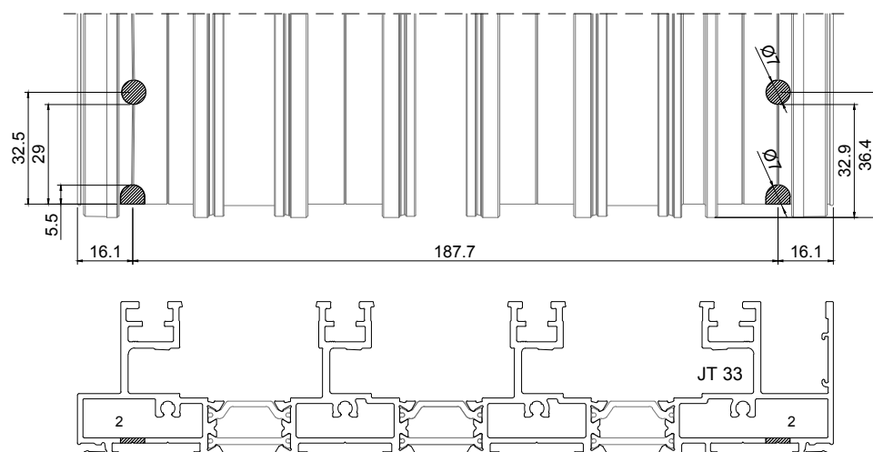
1 - ESQUADRO | CORNER CLEAT | ÉQUERRE JT 12x9.5
