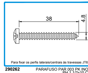
290262 PARAFUSO PAR 003 PK INOX PH 1 1/2x10 CQ
