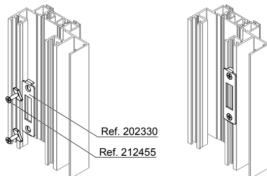
FERRAGEM 1 PONTO/MULTIPONTO ALU
