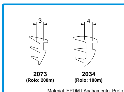
208199 JUNTA DE CUNHA 2073 208195 JUNTA DE CUNHA 2034
