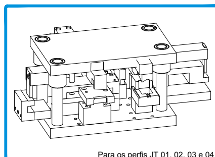
408061 CORTANTE JT - AROS FR
