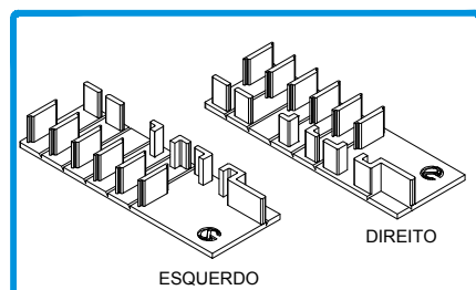
212223 CONJ. TOPOS INFERIORES RENOVARIO
