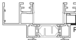
Corte | Cut | Coupe D-D
