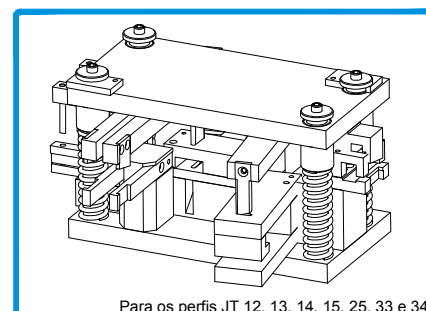
408062 CORTANTE JT - AROS PT
