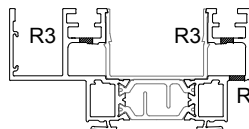
Corte | Cut | Coupe A-A
