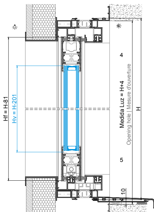
Aberto | Open | Ouvert
