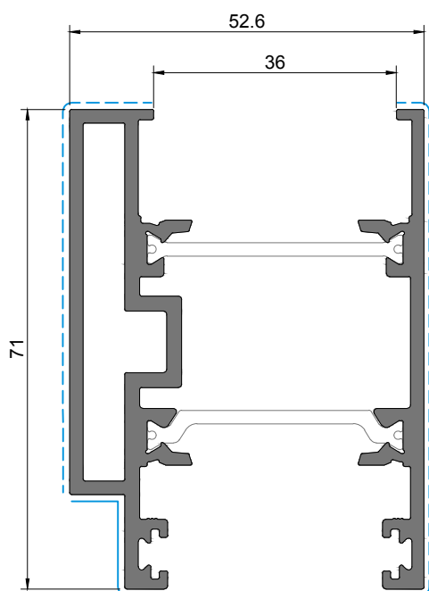
JT 68 Perfil lateral Lateral profile | Profilé latéral (Sacadas) (Full height windows) (Porte-fenêtres)
