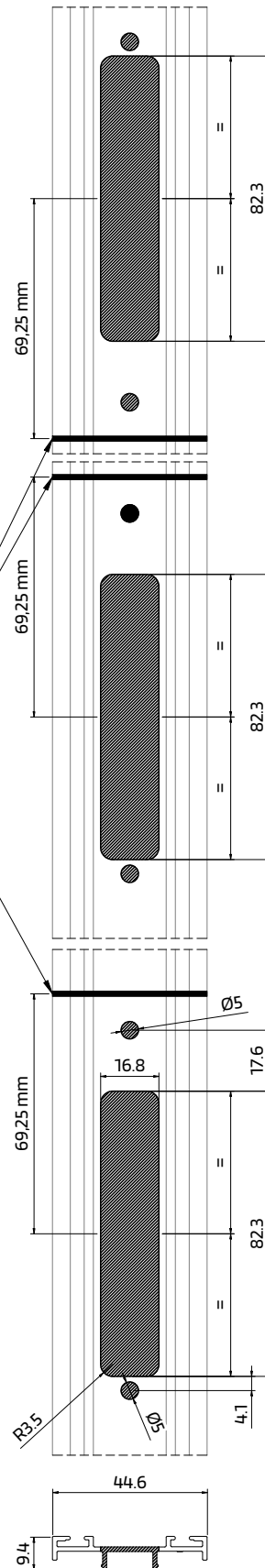
SO 40 Perfil testa fechadura Lock plate profile Profilé plaque pour serrure
