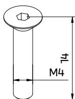
290473 PARAFUSO DIN7991 M4x14 INOX A2
