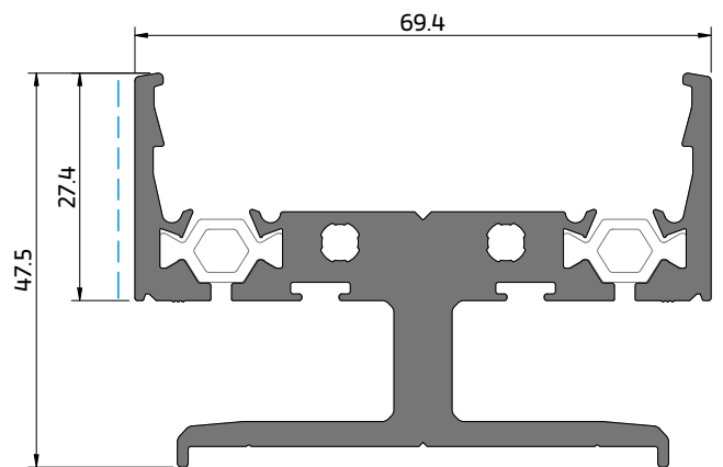
OS 28 Perfil móvel para soleira oculta Concealed sill mobile profile Profilé mobile pour seuil caché
