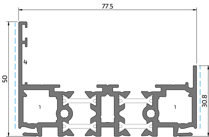
VO 34 Soleira 1-rail 1-rail Sill | Seuil 1-rail
