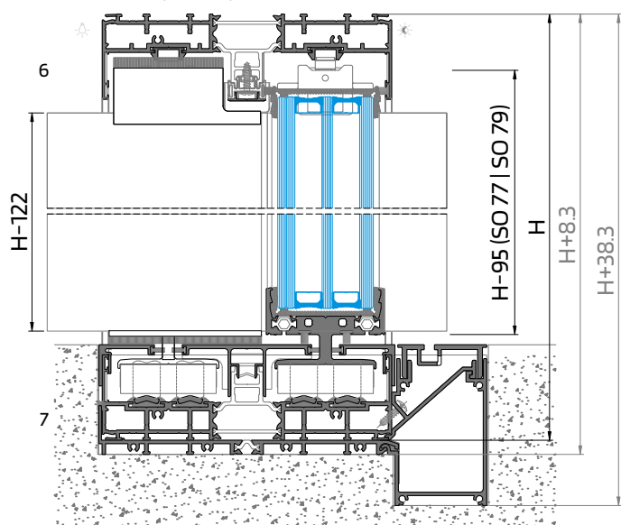
PERFIL | PROFILE | PROFILÉ - OS 28
