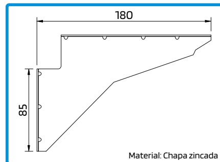
230317 SUPOORTE FIXAÇÃO 180MM Material: Chapa zincada
