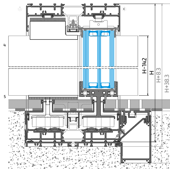
PERFIL | PROFILE | PROFILÉ - OS 38
