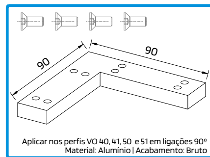
212966 CONJ. UNIÃO CANTO 90° OS-V3
