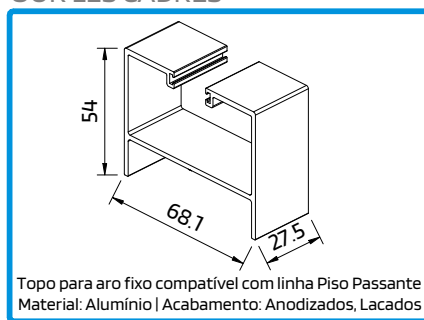
210303 TOPO ARO FIXO SOLEIRA OCULTA N°6 OS-T
