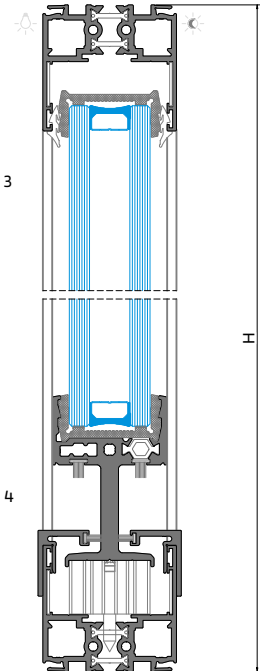
PERFIL | PROFILE | PROFILÉ - OS 38
