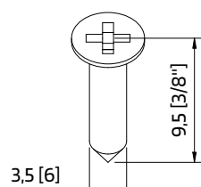
290144 PARAF. DIN7982 PH 3,5x9,5 INOX A2
