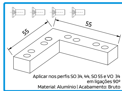
212968 CONJ. UNIÃO CANTO 90° 1-RAIL OS-V3
