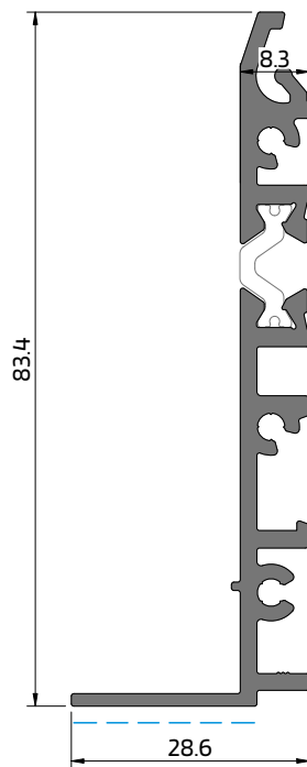
SO 85 Soleira 1-rail para caleira 1-rail Sill for drainage gutter Seuil 1-rail pour gouttière de sol
