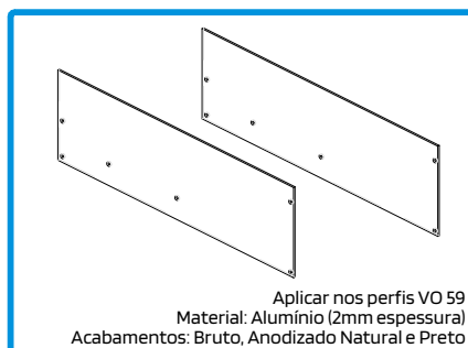
212446 CONJ. TOPOS P/ VO 59
