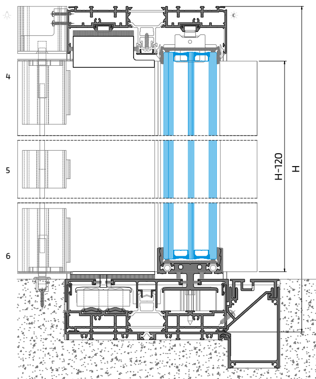
PERFIL | PROFILE | PROFILÉ - OS 28
