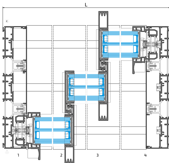
PERFIL | PROFILE | PROFILÉ - OS 28
