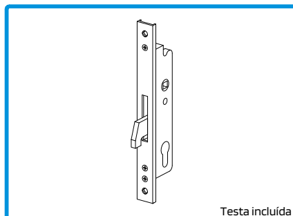
201201 FECHADURA OS MONOPONTO TESTA U
