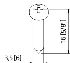
290729 PARAF PKI PH 5/8x6 CQ
