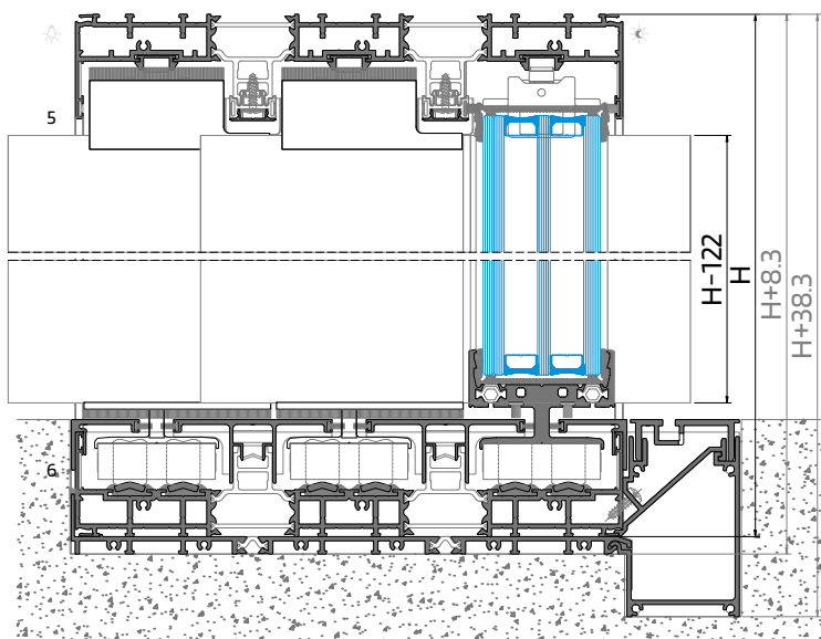
PERFIL | PROFILE | PROFILÉ - OS 28
