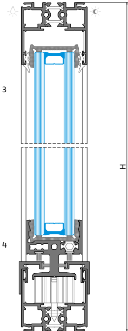
PERFIL | PROFILE | PROFILÉ - OS 28
