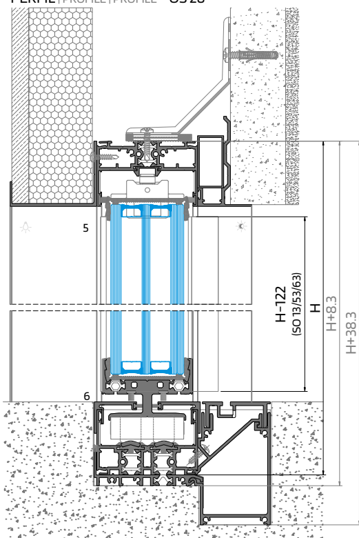
PERFIL | PROFILE | PROFILÉ - OS 28
