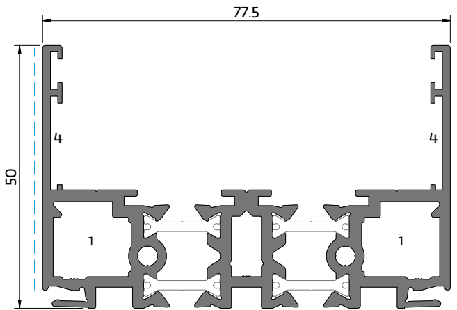
SO 34 Soleira 1-rail 1-rail Sill | Seuil 1-rail
