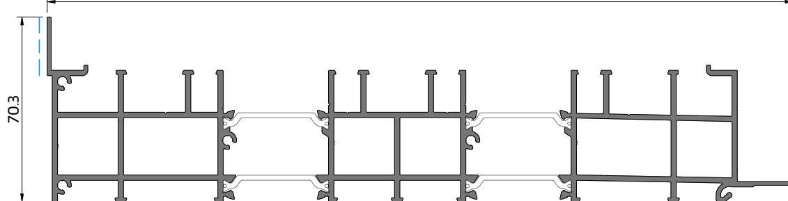
VO 59 - (Esc. | Scl. | Éch.: 1/2)
