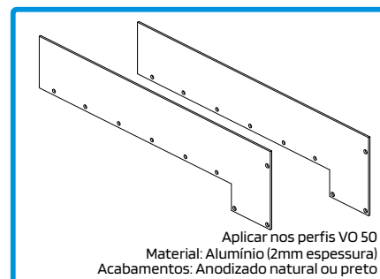
212211 CONJ. TOPOS CALEIRA/SOLEIRA OS-T 3-RAIL
