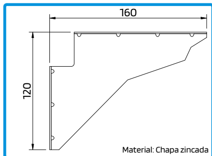
230316 SUPOORTE FIXAÇÃO 160MM Material: Chapa zincada
