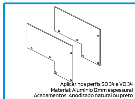
212209 CONJ. TOPOS CALEIRA/SOLEIRA OS-T 1-RAIL
