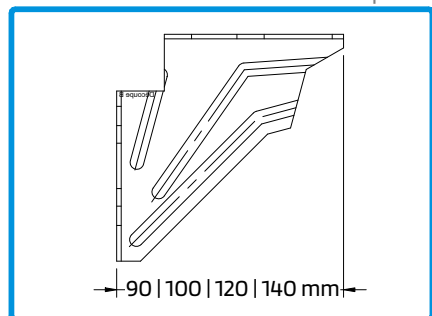
230309 SUPOORTE FIXAÇÃO 90mm 230014 SUPOORTE FIXAÇÃO 100mm 230019 SUPOORTE FIXAÇÃO 120mm 230308 SUPOORTE FIXAÇÃO 140mm
