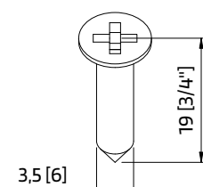
290135 PARAF. DIN7982 PH 3,5x19 INOX A2
