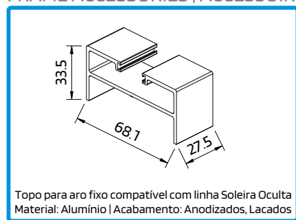
210302 TOPO ARO FIXO SOLEIRA OCULTA N°5 OS-T
