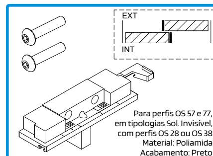
210980 TOPO CENTRAL INV. Nº17 OS-T SOL. OCULTA ESQ
