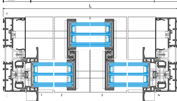
PERFIL | PROFILE | PROFILÉ - OS 28
