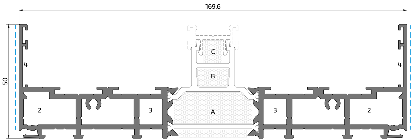
VO 40 soleira 2-rail 2-rail sill | seuil 2-rail
