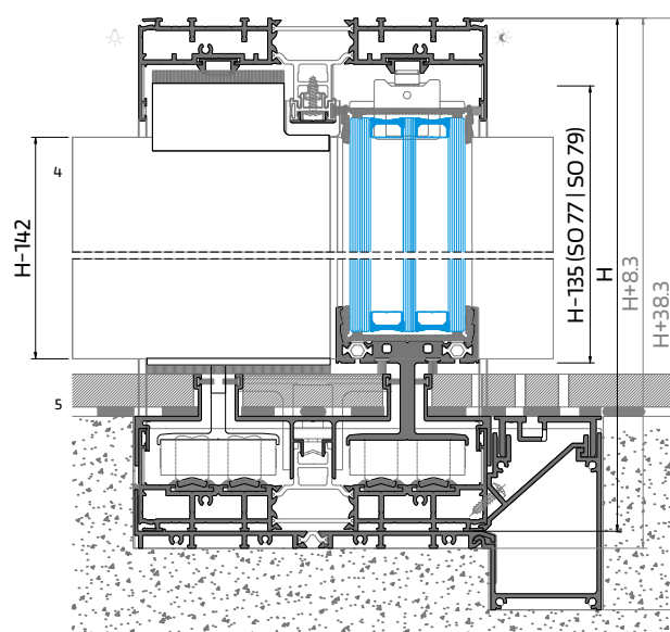
PERFIL | PROFILE | PROFILÉ - OS 38
