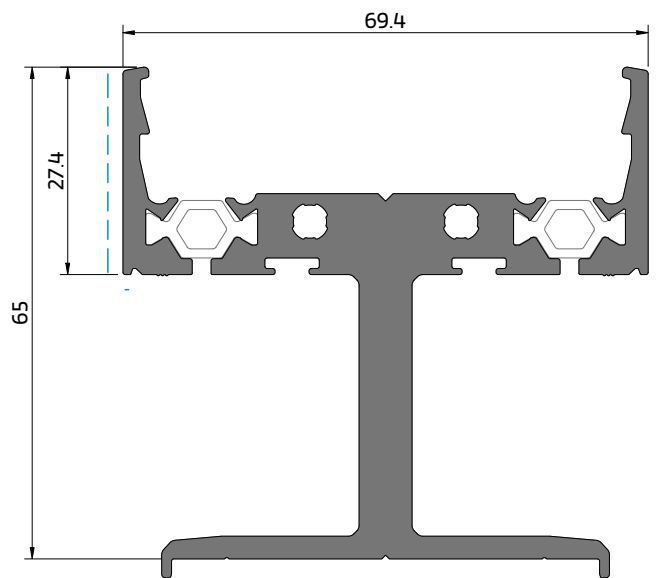
OS 38 Perfil móvel para soleira oculta Concealed sill mobile profile Profilé mobile pour seuil caché
