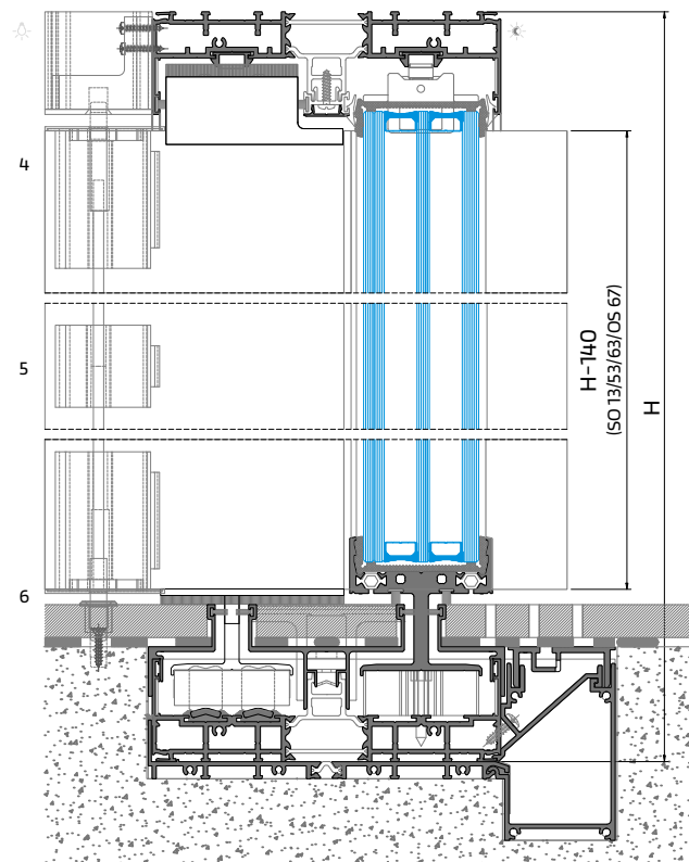
PERFIL | PROFILE | PROFILÉ - OS 38
