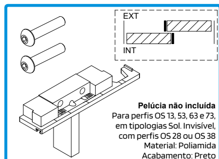
210984 TOPO CENTRAL Nº15 OS-T SOL. OCULTA ESQ
