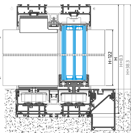
PERFIL | PROFILE | PROFILÉ - OS 28
