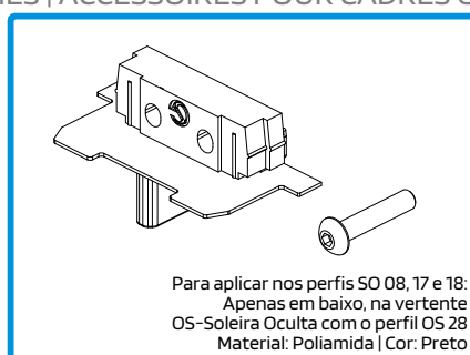
210190 TOPO LATERAL INF. 20MM N°19 OS-V3 SOL. INVIS.
