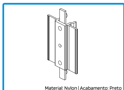
215046 PEÇA AJUSTE FECHO LATERAL OS TRIPLE N°4
