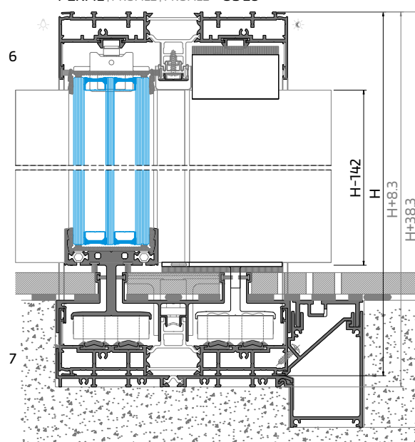
PERFIL | PROFILE | PROFILÉ - OS 28
