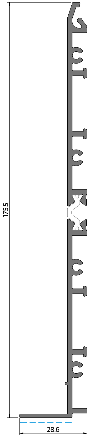
SO 86 Soleira 2-rail para caleira 2-rail Sill for drainage gutter Seuil 2-rail pour gouttière de sol
