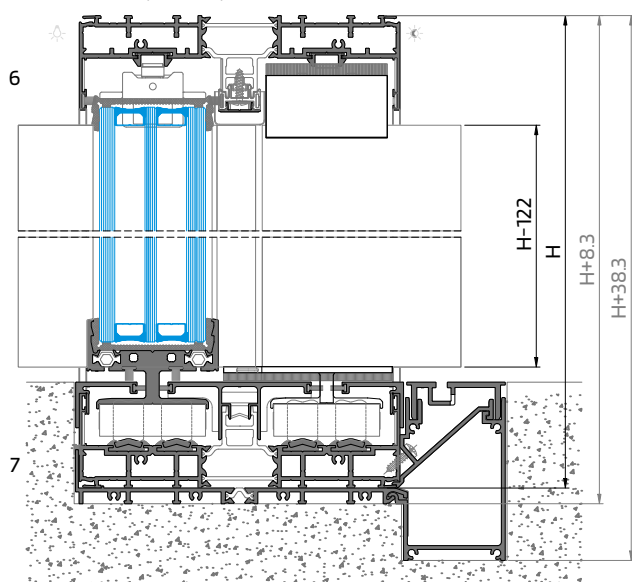
PERFIL | PROFILE | PROFILÉ - OS 28
