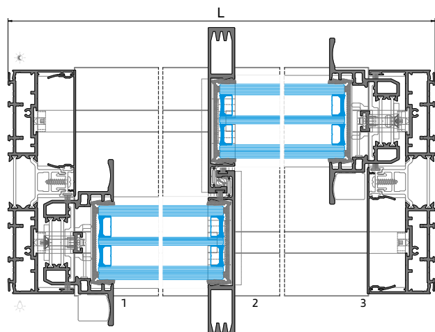
PERFIL | PROFILE | PROFILÉ - OS 28
