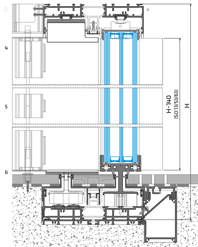
PERFIL | PROFILE | PROFILÉ - OS 28
