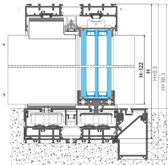
PERFIL | PROFILE | PROFILÉ - OS 28
