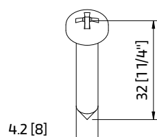
290704 PARAF PKI 11/4X8 CQ
