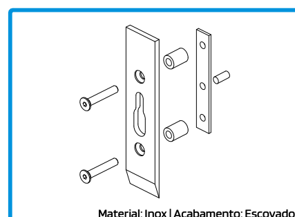
280049 TESTA LARGA OS-TRIPLE / FECHO OS N°2
