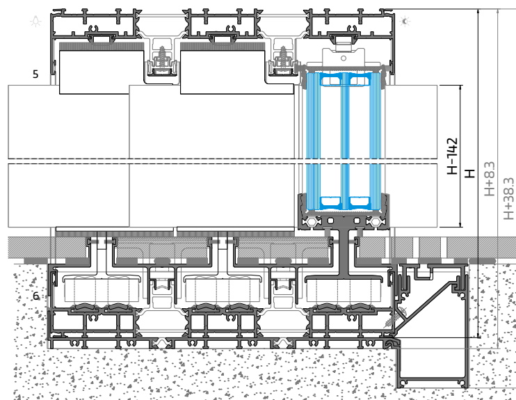
PERFIL | PROFILE | PROFILÉ - OS 38
