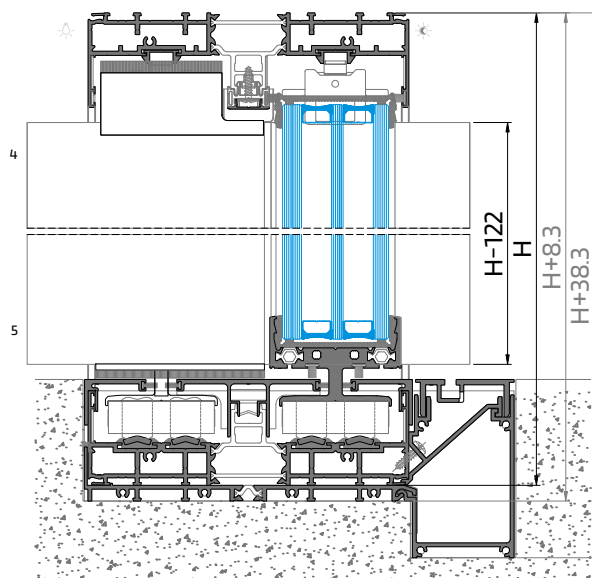
PERFIL | PROFILE | PROFILÉ - OS 28
