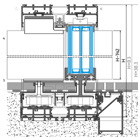
PERFIL | PROFILE | PROFILÉ - OS 38
