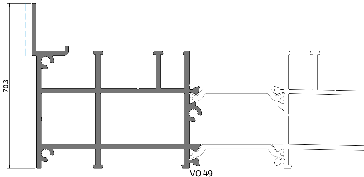
VO 49 - (Esc. | Scl. | Éch.: 1/2)
