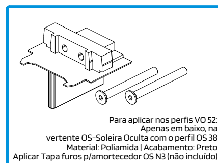
210306 TOPO LAT. INF. 40MM N°26 OS-T SOL. INVIS. FECH.
