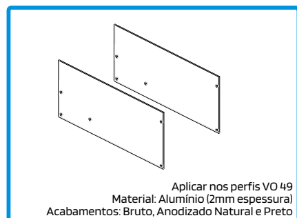
212445 CONJ. TOPOS P/ VO 49
