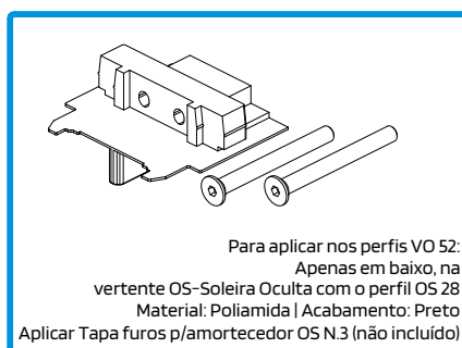
210305 TOPO LAT. INF. 20MM N°25 OS-T SOL. INVIS. FECH.
