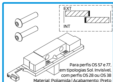
210981 TOPO CENTRAL INV. Nº17 OS-T SOL. OCULTA DIR
