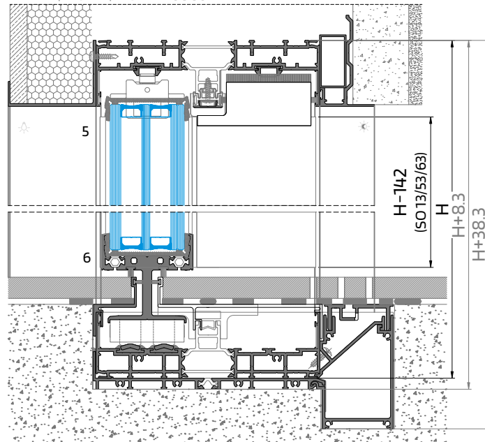
PERFIL | PROFILE | PROFILÉ - OS 38
