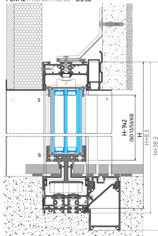
PERFIL | PROFILE | PROFILÉ - OS 38
