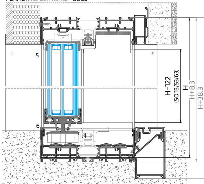
PERFIL | PROFILE | PROFILÉ - OS 28
