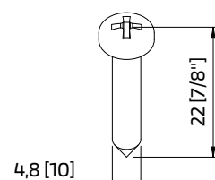
290020 PARAFUSO PAR 006 7/8x10 CQ
