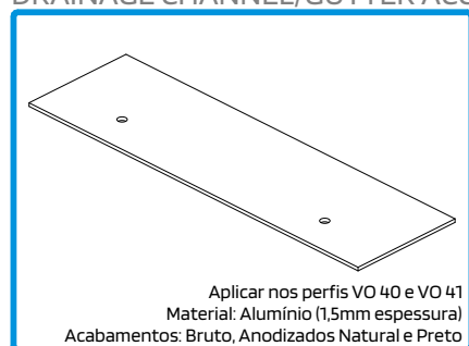
210199 TOPO PARA VO40/VO41
