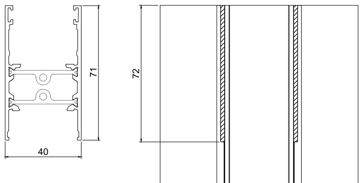
JT 63 Travessa superior Upper transom | Traverse supérieur
