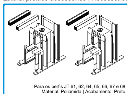
212199 CONJ. TOPOS LAT. JT N°1 Para os perfis JT 61, 62, 64, 65, 66, 67 e 68 Material: Poliamida | Acabamento: Preto
