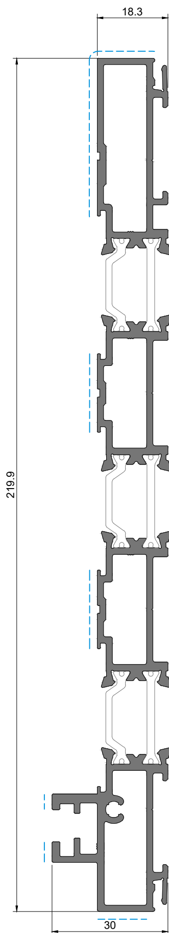
JT 39 Ombreira 90° 4rail 4rail 90° jamb | Jambage 90° 4rail
