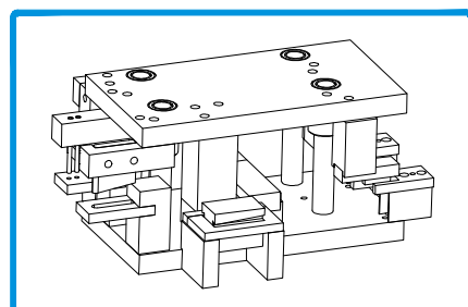
408060 CORTANTE JT - FOLHAS
