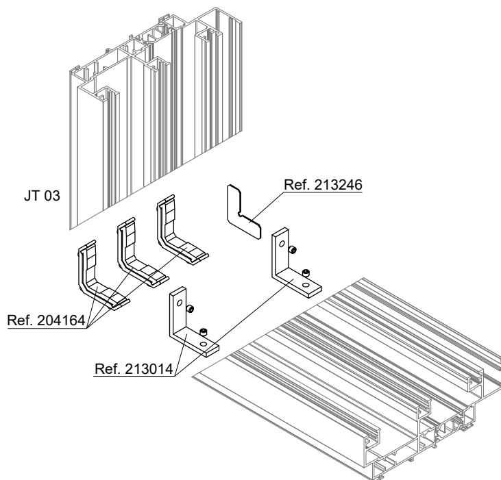
213014 CANTO ALINHAMENTO JT
