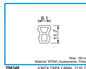
208348 JUNTA TAPA CANAL 2116 JT
