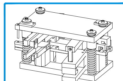
408062 CORTANTE JT - AROS PT
