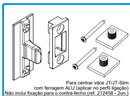
212291 CONJ. CENTRADOR P/ FERR. ALU PERFIL LIG.
