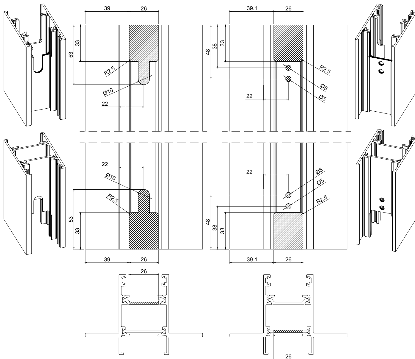
JT 65 Perfil Lateral Lateral profile | Profilé latéral
