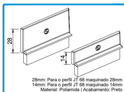
210288 TOPO LATERAL JT68 28MM 210289 TOPO LATERAL JT68 14MM 28mm: Para o perfil JT 68 maquinado 28mm 14mm: Para o perfil JT 68 maquinado 14mm Material: Poliamida | Acabamento: Preto
