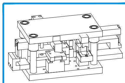
408061 CORTANTE JT - AROS FR
