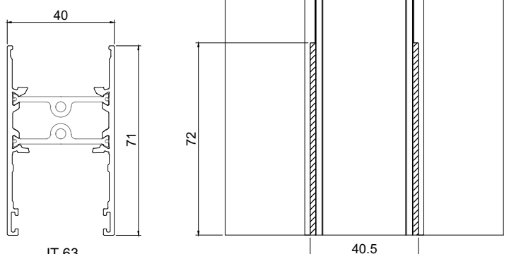
JT 63 Travessa inferior Lower transom | Traverse inférieur
