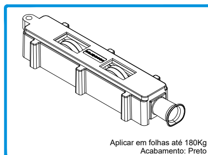
205129 CARRINHO JT 180KG Aplicar em folhas até 180Kg Acabamento: Preto
