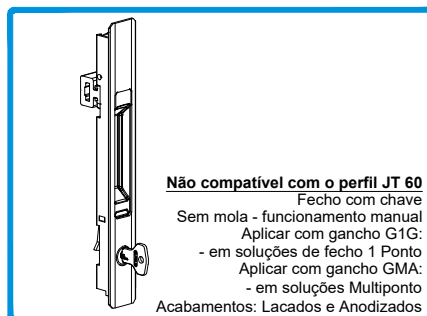
201383 FECHO DE EMBUTIR C/ CHAVE R2053IX
