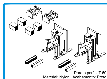
212131 CONJ. TOPOS LATERAL JT-SLIM Para o perfil JT 60 Material: Nylon | Acabamento: Preto
