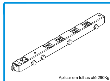
205202 CARRINHO JT-SLIM HEAVY DUTY Aplicar em folhas até 290Kg
