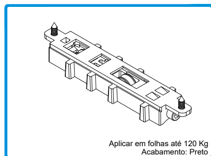
205000 CARRINHO JT-SLIM Aplicar em folhas até 120 Kg Acabamento: Preto
