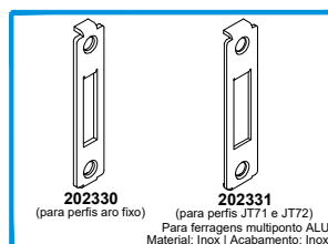
202330 CONTRA-FECHO ALU 202331 CONTRA-FECHO Nº2 2F/90º ALU
