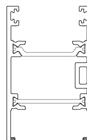
JT 67 Perfil Lateral Lateral profile Profilé latéral
