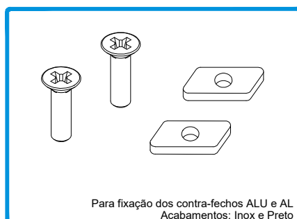
212455 CONJ. FIX. CONTRA-FECHO AL MULTIP. JT
