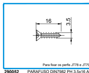
290052 PARA FUSO DIN7982 PH 3,5x16 A2
