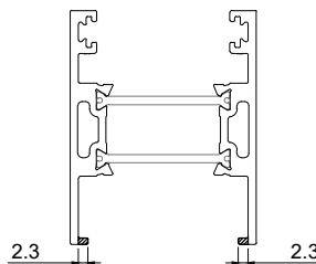
JT 60 Perfil Lateral Lateral profile | Profilé latéral
