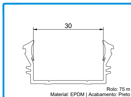
208478 JUNTA VIDRO U 1030 CX 30MM JT
