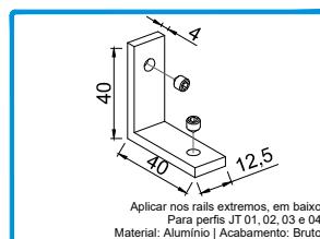
213014 CANTO ALINHAMENTO JT
