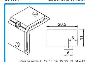
204153 ESQUADRO JT 11x20.5
