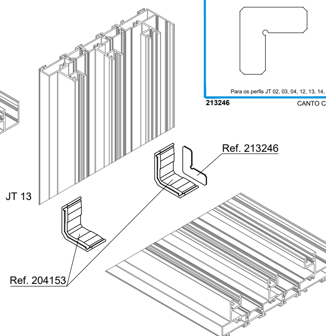
204153 ESQUADRO JT 11x20.5
