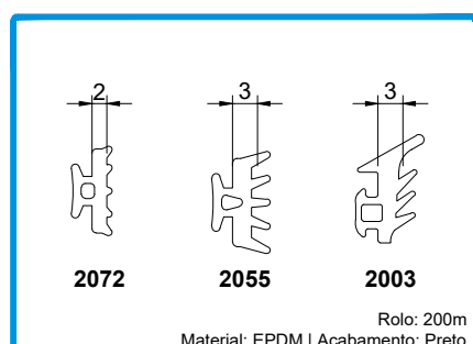
208224 JUNTA VD 2072 208289 JUNTA DE BATEENTE 2055 208350 JUNTA DE VEDAÇÃO EXT. 2003
