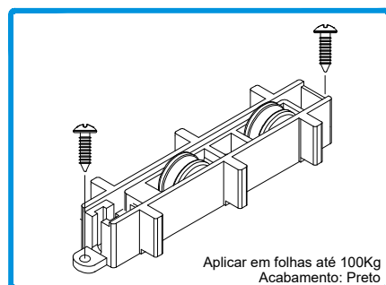
205108 CARRINHO JT 100KG Aplicar em folhas até 100Kg Acabamento: Preto
