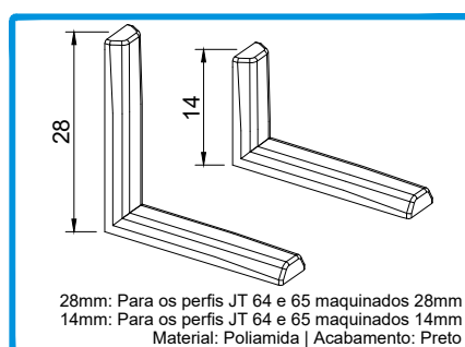
210239 TOPO JT64/JT65 28MM 210240 TOPO JT64/JT65 14MM 28mm: Para os perfis JT 64 e 65 maquinados 28mm 14mm: Para os perfis JT 64 e 65 maquinados 14mm Material: Poliamida | Acabamento: Preto
