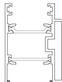
JT 68 Perfil Lateral Lateral profile Profilé latéral
