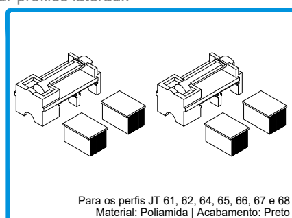
212230 CONJ. TOPOS INTERIORES LAT. JT Para os perfis JT 61, 62, 64, 65, 66, 67 e 68 Material: Poliamida | Acabamento: Preto
