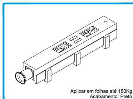
205111 CARRINHO JT-SLIM 180KG Aplicar em folhas até 180Kg Acabamento: Preto
